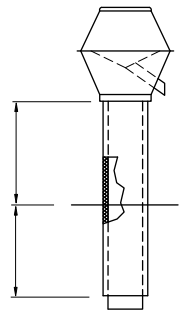
Tipo ARI per tetto piano
