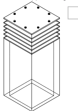
CEID doppelwandig, 50 mm isoliert
