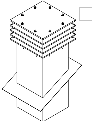
CE-S mit Tablett für Schrägdach
